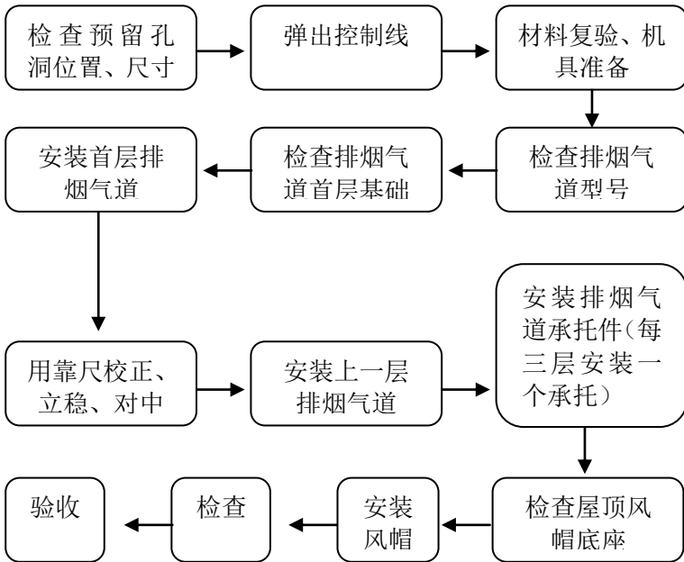
图 6.1.6 施工工艺流程
